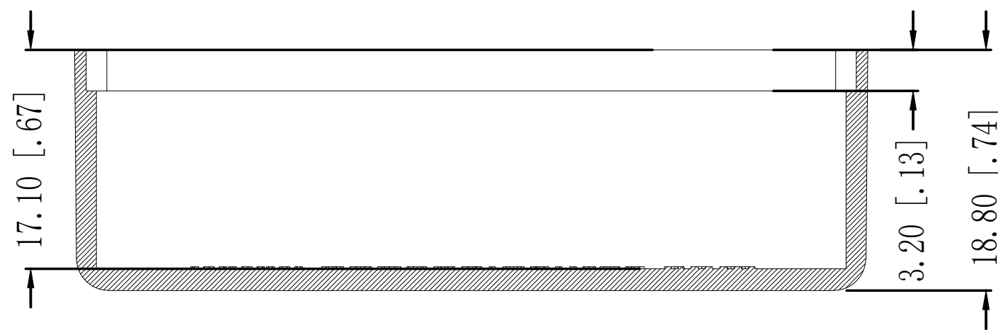
SECTION A-A
