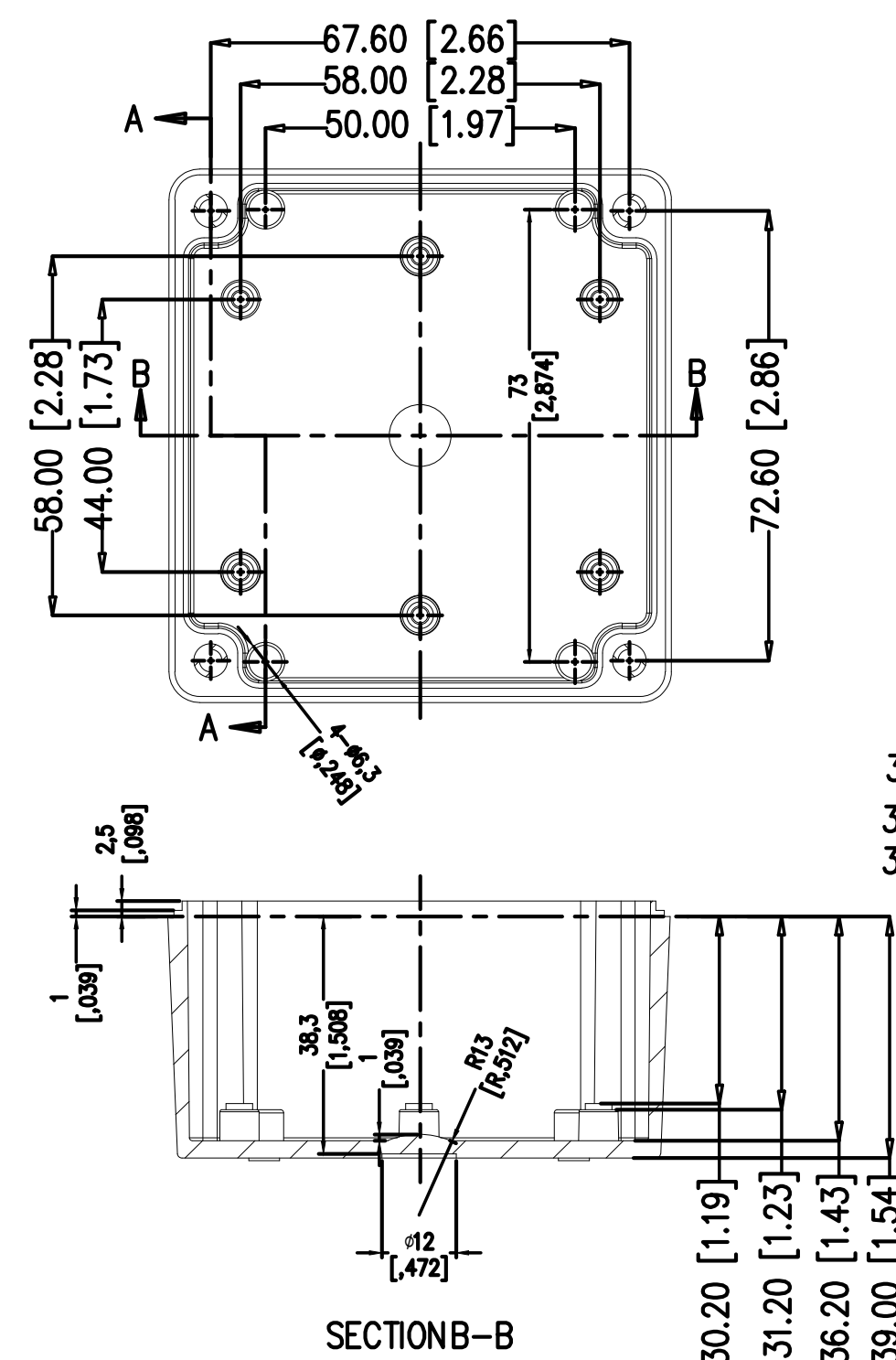
BEN-20-BOTTOM
